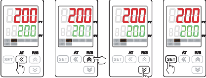
短按“SET”键SV值闪烁 短按“AT”键增加SV值 短按“R/S”键减少SV值 短按“SET”键保存SV值
