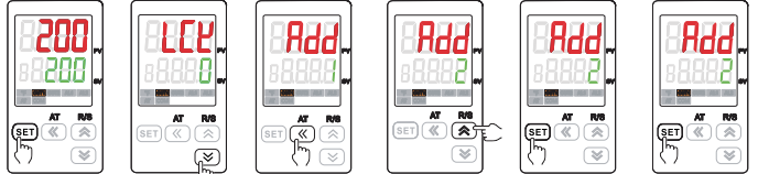
长按“SET”键 3秒进入常用菜单 短按“AT”键 切换菜单 短按“R/S”键 修改参数 短按“SET”键 保存参数 短按“AT”键 修改参数 短按“R/S”键 保存参数 长按“SET”键 3秒退出菜单
