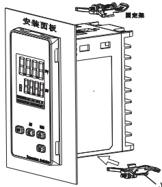
安装示意图
