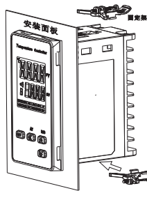
安装示意图
