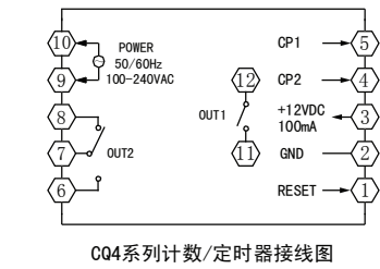
CQ4系列计数/定时器接线图
