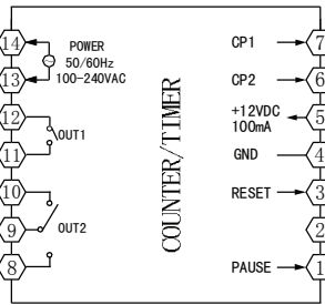
CQ7系列计数/定时器接线图
